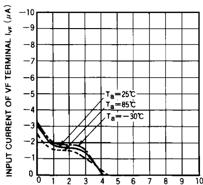
VF TERMINAL VOLTAGE V_{VF} (V)
